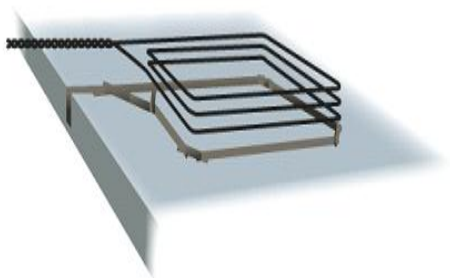
Εικόνες 4.11 και 4.12: Απλός επαγωγικός βρόχος σε σχεδιαστική απεικόνιση (αριστερά) και μετά την εγκατάσταση (δεξιά)
