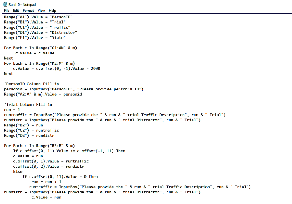
Εικόνα 4.17: Εντολές script
