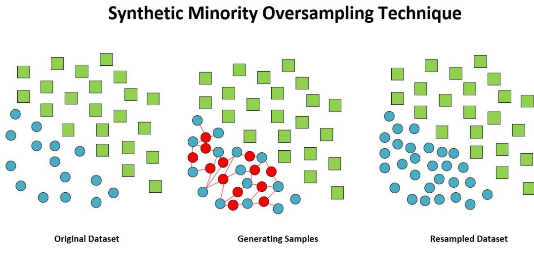
Γράφημα 3.2: SMOTE: Synthetic Minority Oversampling Technique Πηγή: Medium (2022)
