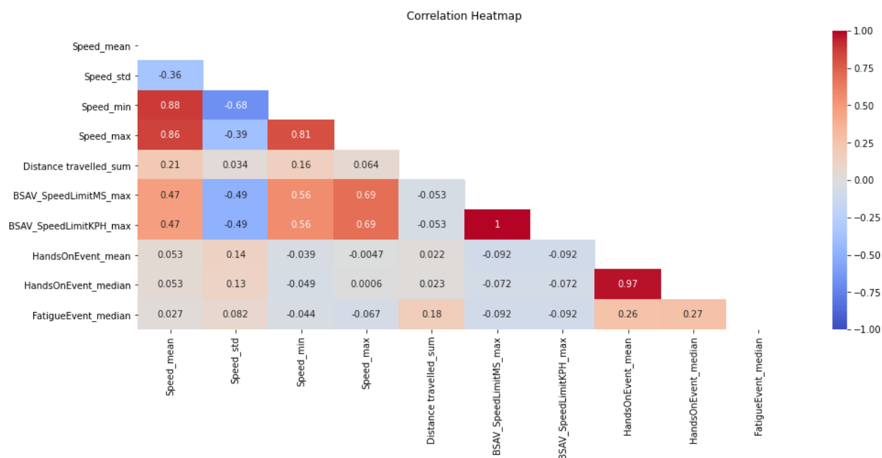
Γράφημα 5.1: Συσχέτιση μεταβλητών προς εξέταση
