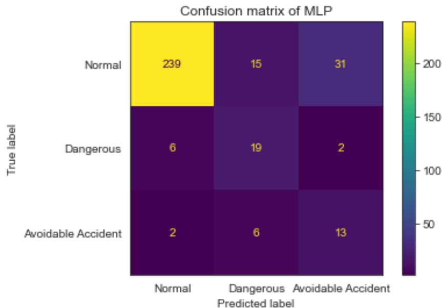
Γράφημα 5.11: Μήτρα σύγχυσης αλγόριθμου MLP
