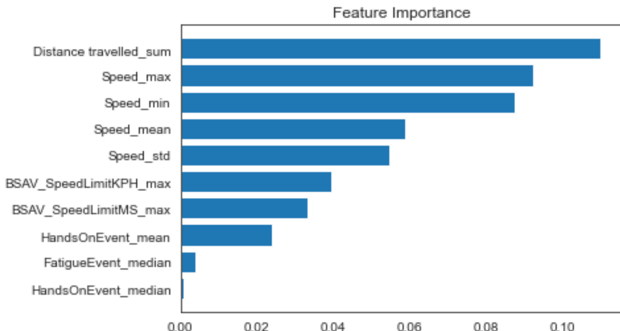
Γράφημα 1: Σημαντικότητα μεταβλητών για την πρόβλεψη του επιπέδου 'Ζώνης Ανοχής Ασφαλείας'
