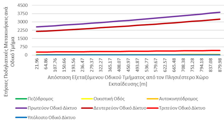
Διάγραμμα 5.4: Απόσταση Εξεταζόμενου Οδικού Τμήματος από τον Πλησιέστερο Χώρο Εκπαίδευσης
