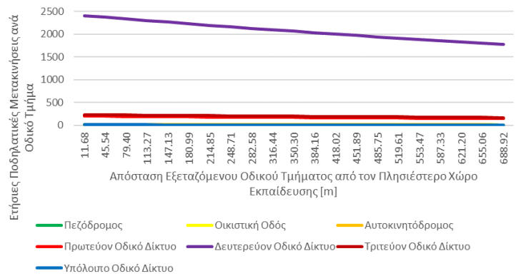
Διάγραμμα 5.10: Απόσταση Εξεταζόμενου Οδικού Τμήματος από τον Πλησιέστερο Χώρο Εκπαίδευσης
