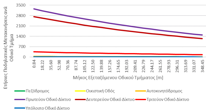
Διάγραμμα 5.2: Μήκος Εξεταζόμενου Οδικού Τμήματος
