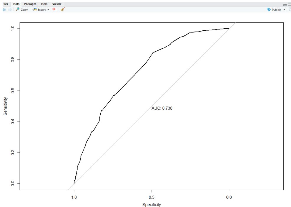
Εικόνα 5.1: Καμπύλη ROC
