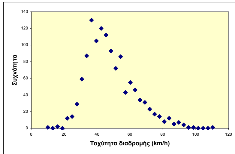
Διάγραμμα 5.1: Κατανομή ταχυτήτων (παράγοντας απόσπασης προσοχής: δύσκολη κλήση).
