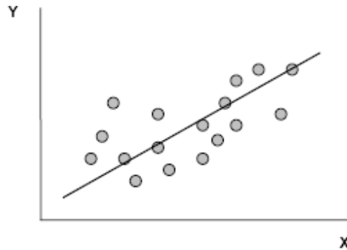
Διάγραμμα 3.1: Ευθεία ελαχίστων τετραγώνων
