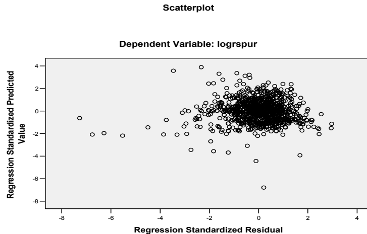
Διάγραμμα 5.35: Συσχέτιση και διασπορά των σφαλμάτων στο μοντέλο της μέσης απόστασης από τον άξονα της οδού που αφορά στη χρήση κινητού τηλεφώνου κατά την οδήγηση (εύκολη κλήση).
