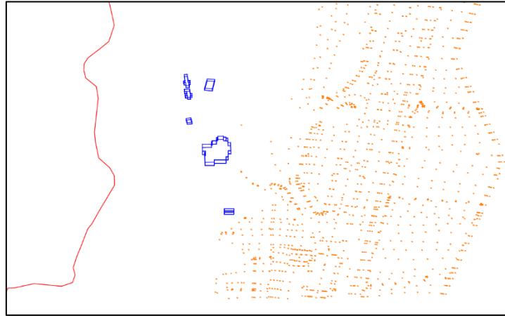
Εικόνα 23. Κτίρια αεροδρομίου Ιωαννίνων στο σχέδιο των ισοϋψών και διαδρόμου.
