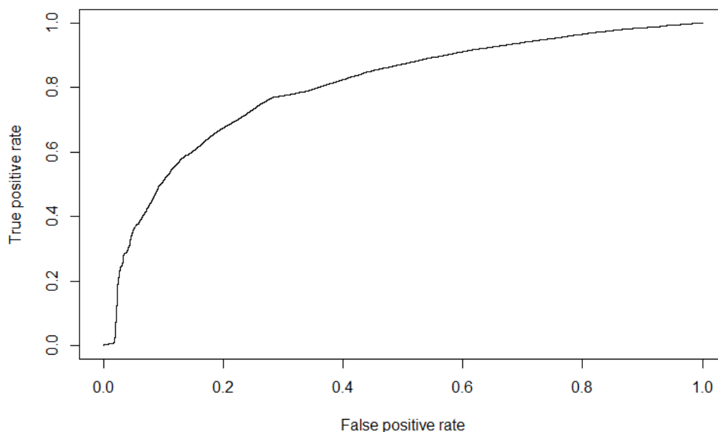
Εικόνα 5.1: Καμπύλη ROC
