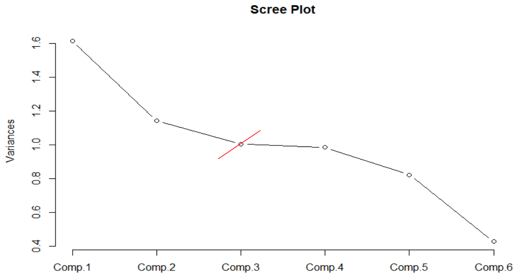
Εικόνα 5.3: Διάγραμμα Διακύμανσης-Συνιστωσών
